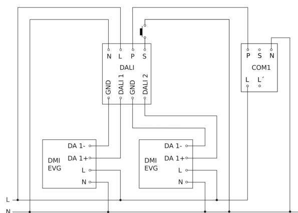
Diagrama electrónico interconexión maestro-maestro
